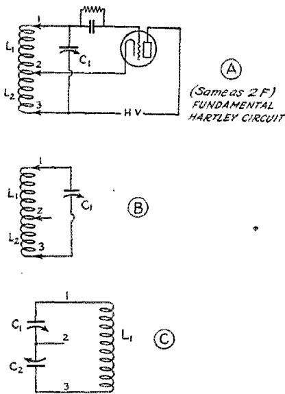
FIG 9A-HARTLEY & COLPITS
