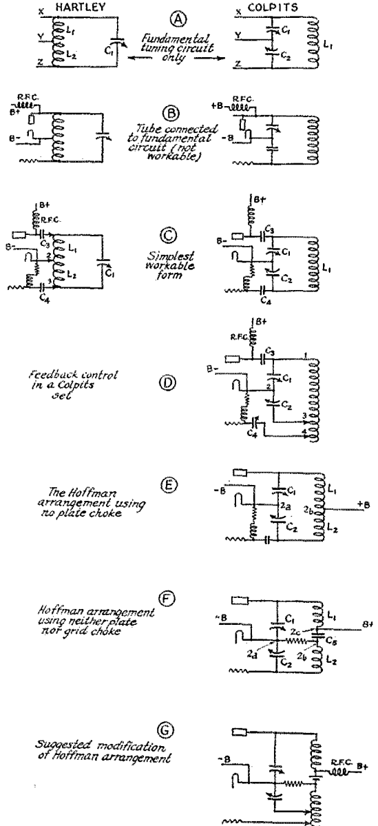
FIG. 10 COLPITS CIRCUITS
